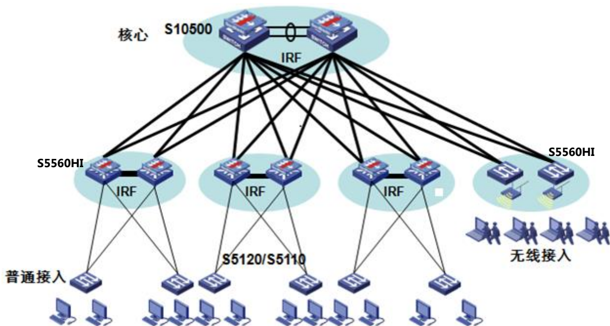
S5560-HI 系列以太网交换机在企业网/园区网汇聚层应用
