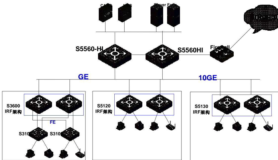
S5560-HI 系列以太网交换机在核心层的应用
