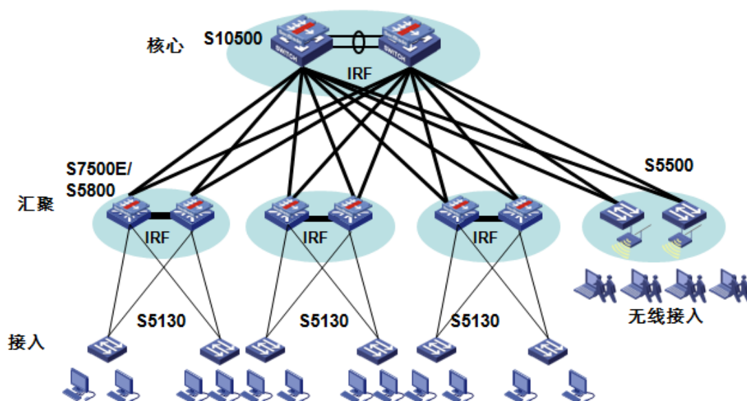
S5130-SI 系列以太网交换机在企业网/园区网汇聚层应用
