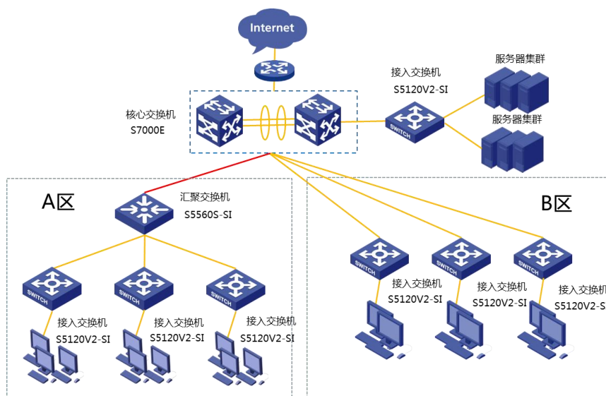
S5120V2-SI 接入交换机应用示意图
