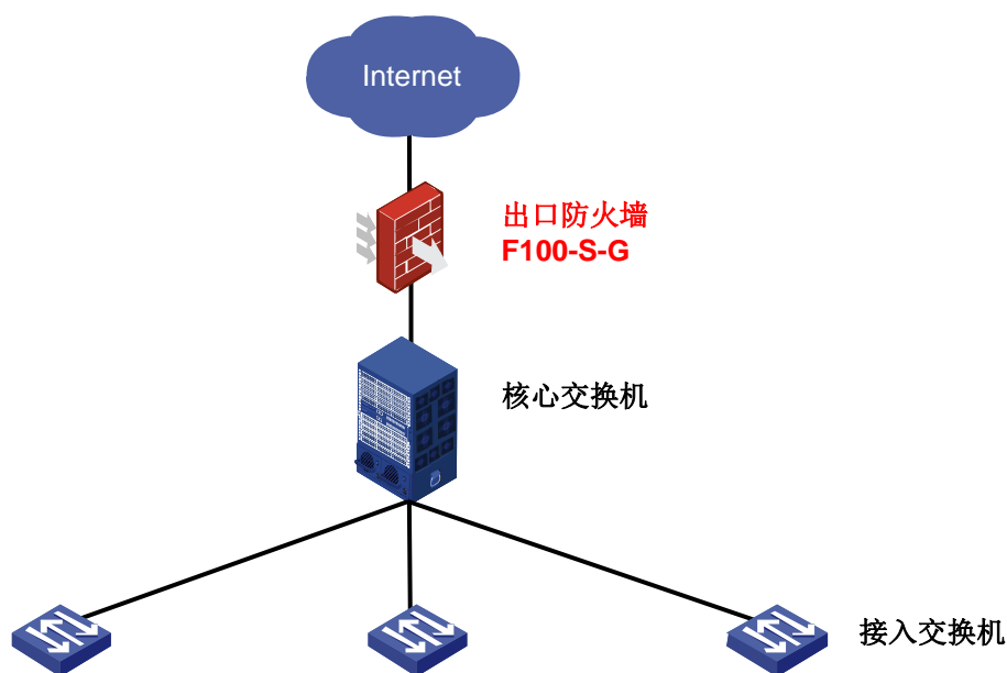
F100-S-G 中小企业 Internet 出口应用示意图
