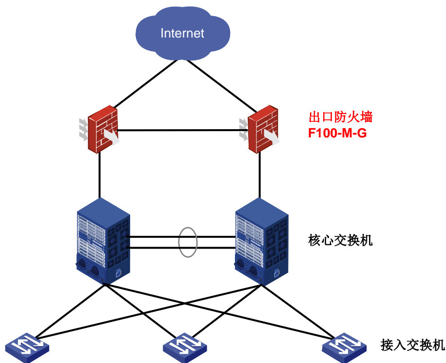
F100-M-G 中小企业 Internet 出口应用示意图
