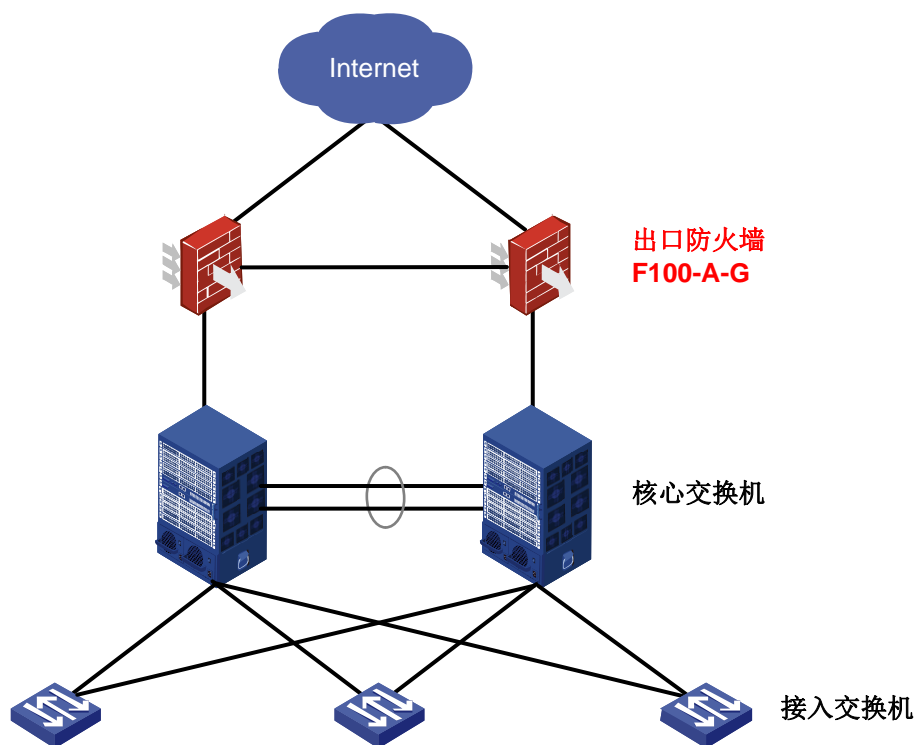
F100-A-G 中小企业 Internet 出口应用示意图
