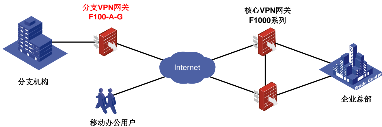
F100-A-G 分支机构互联 VPN 应用示意图
