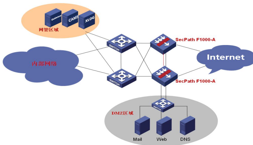
SecPath F1000-A-EI 防火墙应用典型部署图
